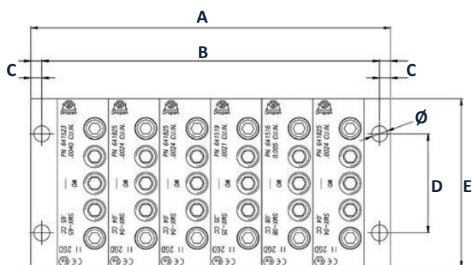
DIMENSIONES SMX
